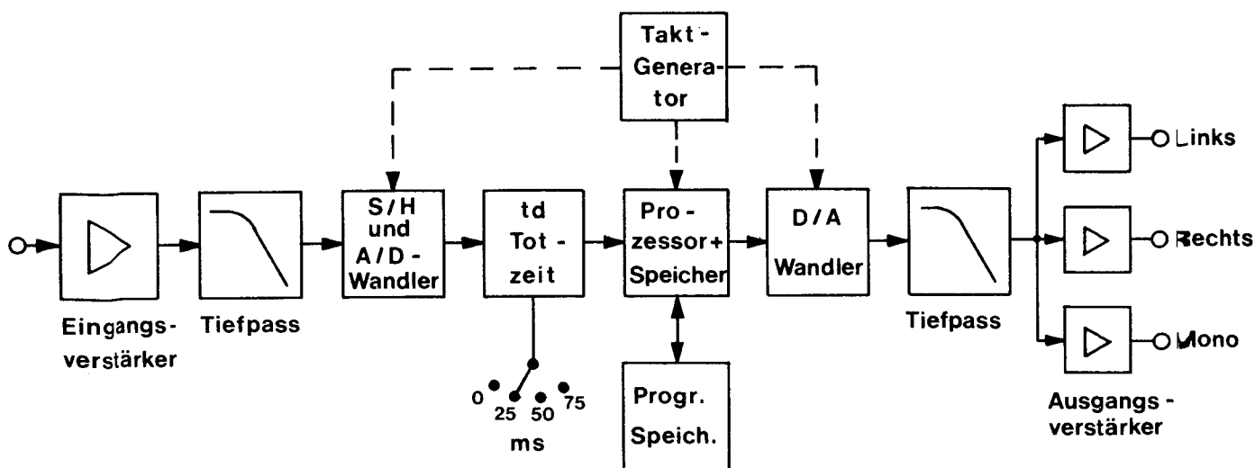
Blockschaltung des digitalen Verarbeitungsprozesses in Betriebsart „Hall“
